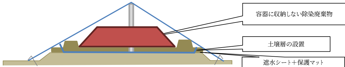
図 2-12 水分を含む除染廃棄物を容器に収納しない場合の汚水流出防止（例）
