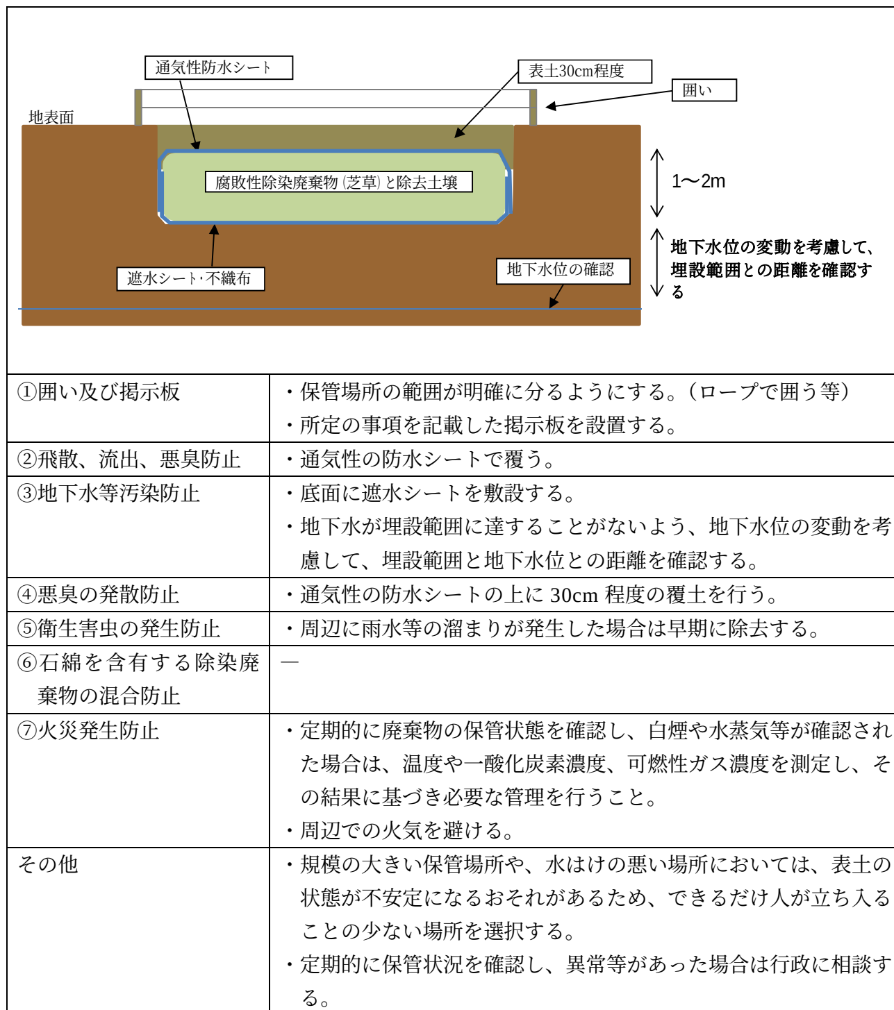
図 2-24 除染廃棄物（芝草）の保管例
