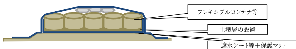
図 2-11 水分を含む除染廃棄物をフレキシブルコンテナに収納した場合の汚水漏出防止（例）
