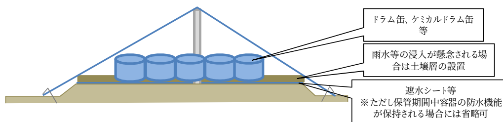
図 2-10 水分の多い除染廃棄物を密閉性の高い容器に収納した場合の汚水漏出防止（例）
