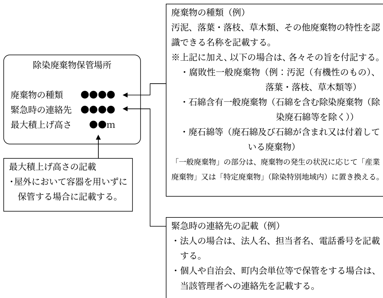
図 2-4 掲示板 (例)
