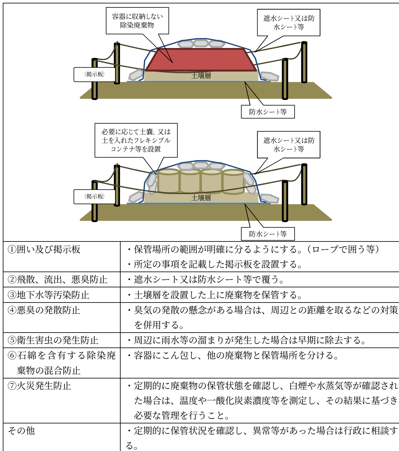
図 2-21 除染廃棄物の保管例（１）
