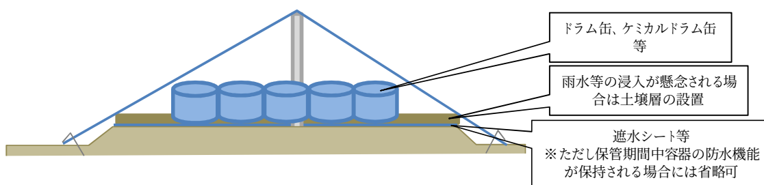
図2-11 水分の多い指定廃棄物を密閉性の高い容器に収納した場合の汚水漏出防止（例）
