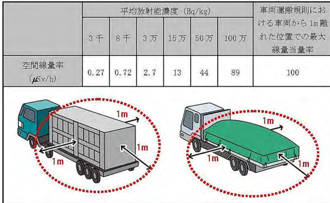
図 2.1.3-10 輸送車両から 1\text{m} の地点における空間線量率の試算例
