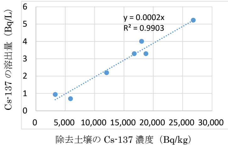
図. 除去土壌（分別後）の溶出試験結果について（検出されたもののみをプロット）
