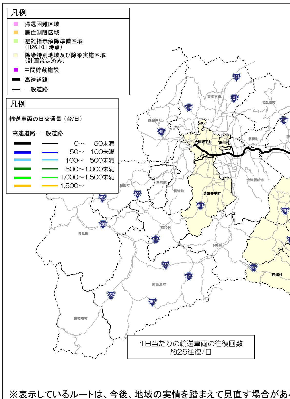
図 7-7 パイロット輸送時「①混雑：輸送車両の日交通量」の試算結果
