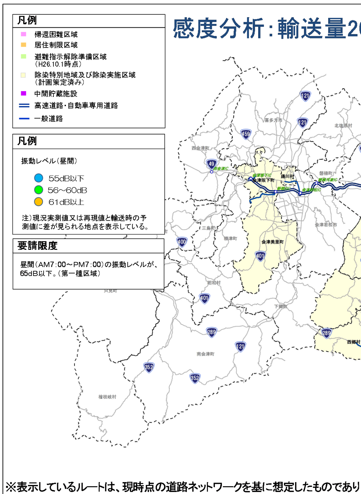
図 9-18 【感度分析：輸送量 20%増】本格輸送時「③生活：振動（昼間）」の試算結果
