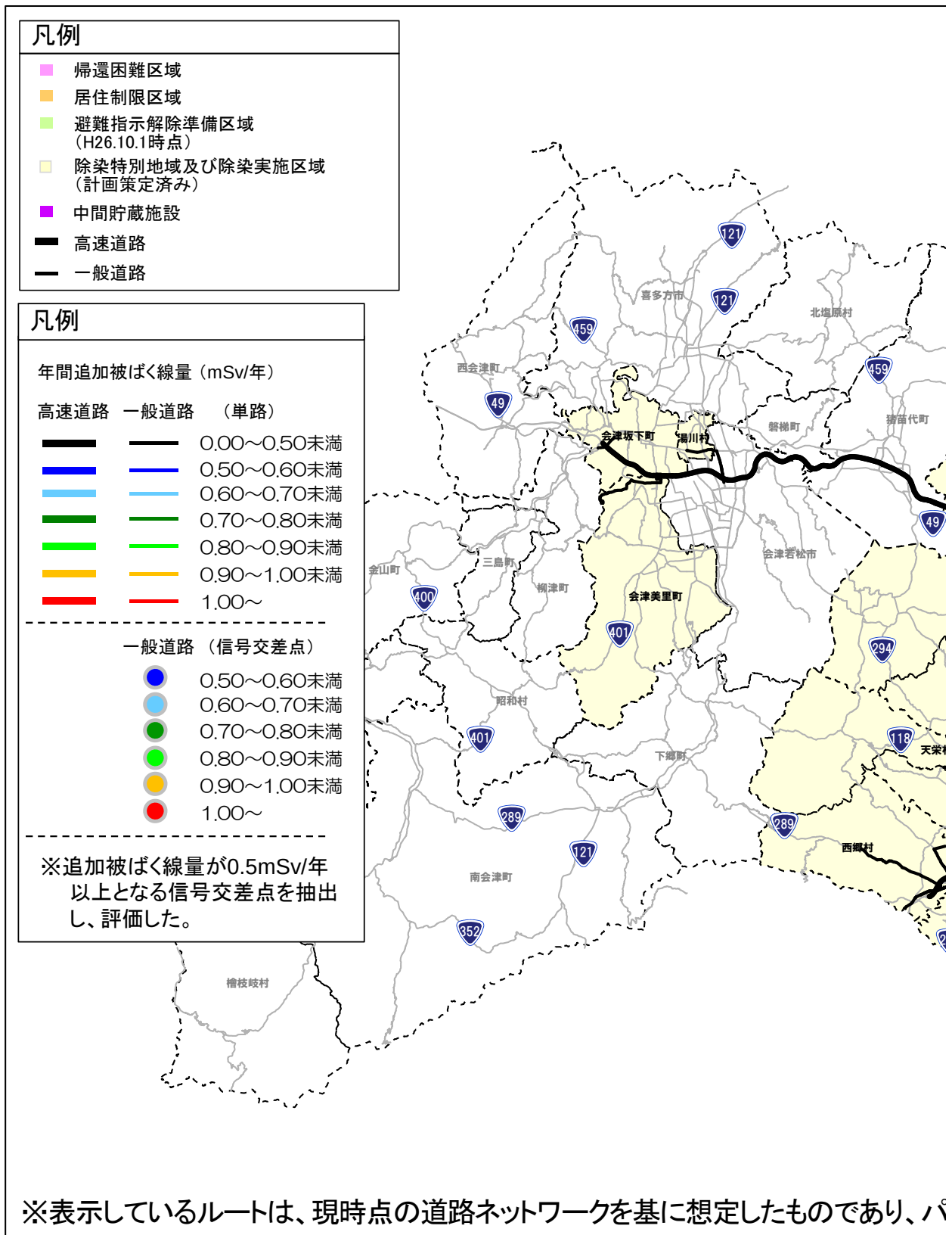
図 9-5 本格輸送時「②被ばく：輸送による公衆の年間追加被ばく線量」の試算結果
