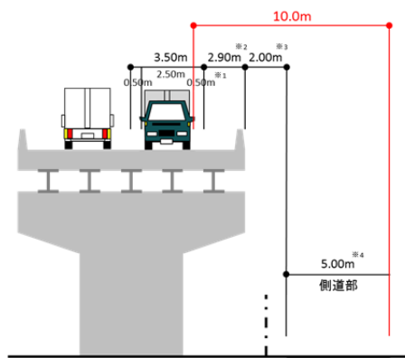
図 7-4 輸送車両側面と高速道路沿道居住者との離隔
