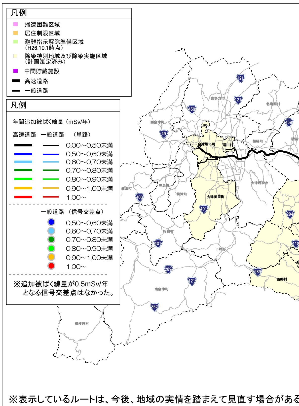
図 7-10 パイロット輸送時「②被ばく：輸送による公衆の年間追加被ばく線量」の試算結果
