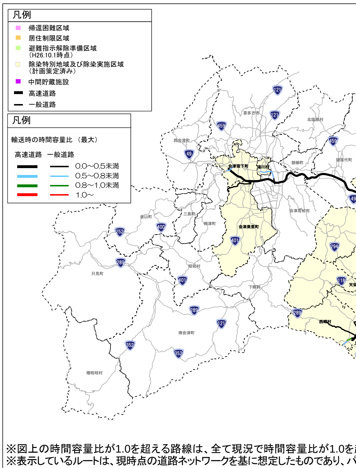
図 9-4 本格輸送時「①混雑：輸送車両の時間容量比 (最大)」の試算結果
