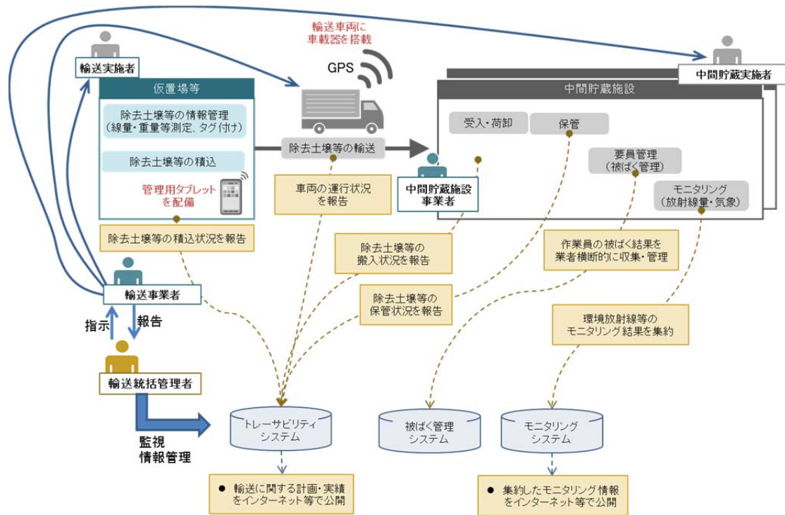
図 4-2 総管理システムの概要
