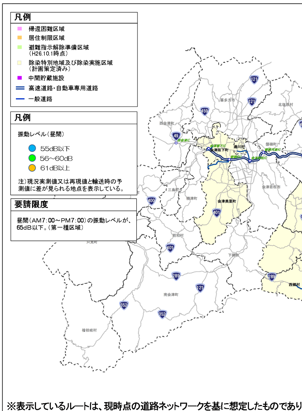
図 9-9 本格輸送時「③生活：振動（昼間）」の試算結果
