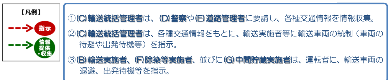
図 5-4 事故車両以外の輸送車両への対応（連絡・指示系統図）
