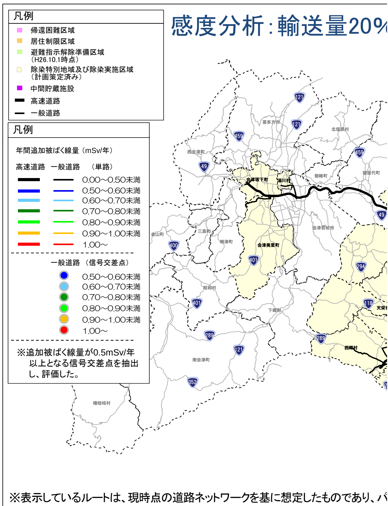
図 9-14 【感度分析：輸送量 20%増】本格輸送時「②被ばく：輸送による公衆の年間追加被ばく線量」の試算結果
