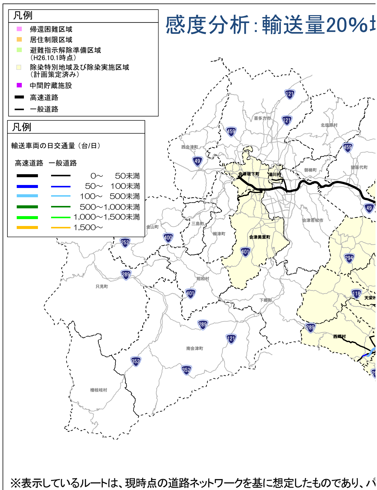
図 9-11 【感度分析：輸送量 20%増】本格輸送時「①混雑：輸送車両の日交通量」の試算結果
