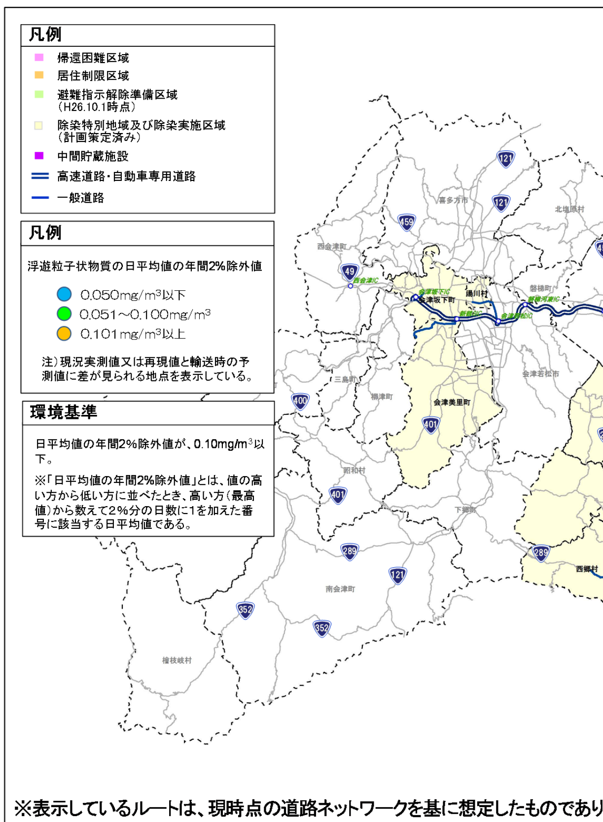
図 9-7 本格輸送時「③生活：浮遊粒子状物質」の試算結果
