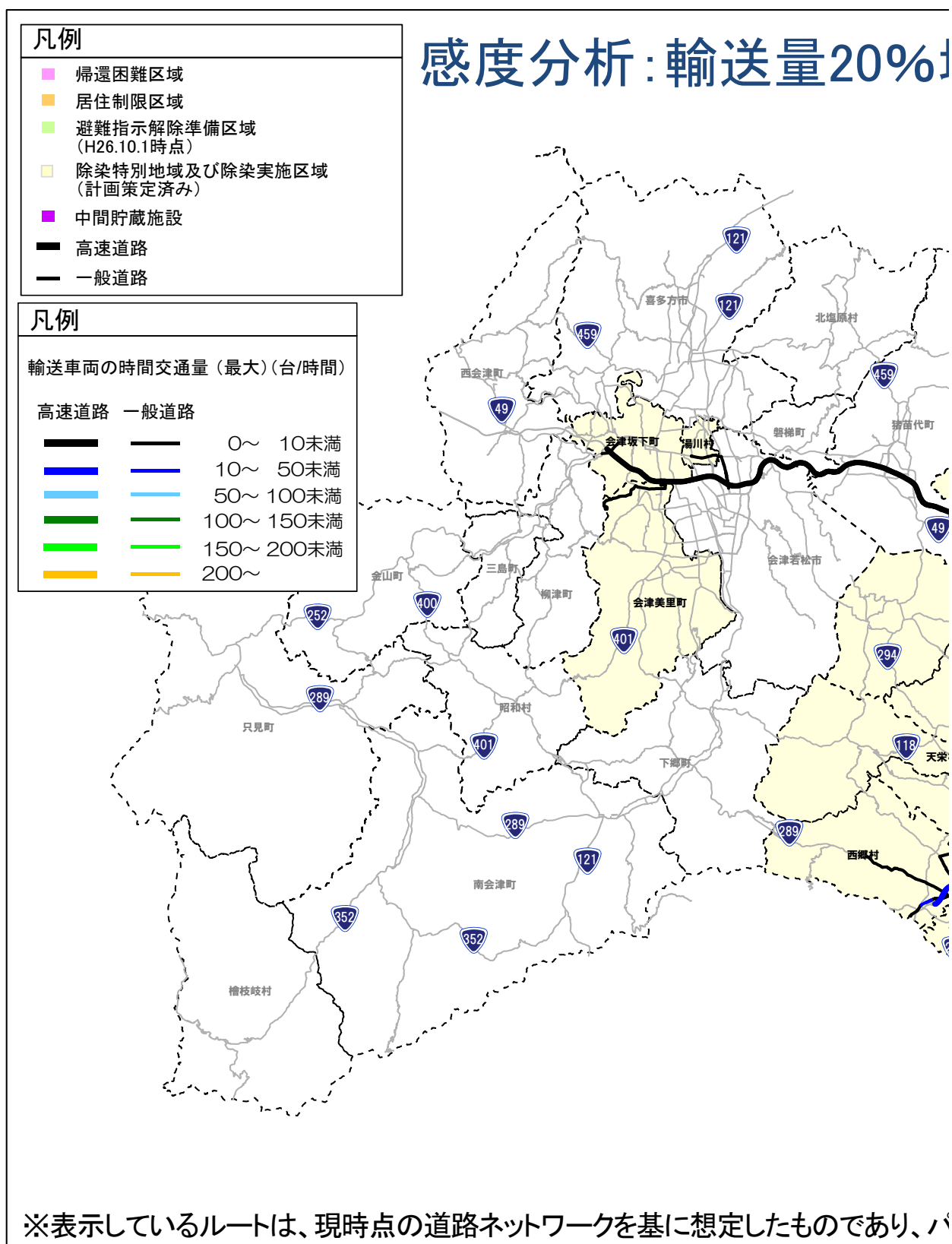
図 9-12 【感度分析：輸送量 20%増】本格輸送時「①混雑：の輸送車両の時間交通量」の試算結果
