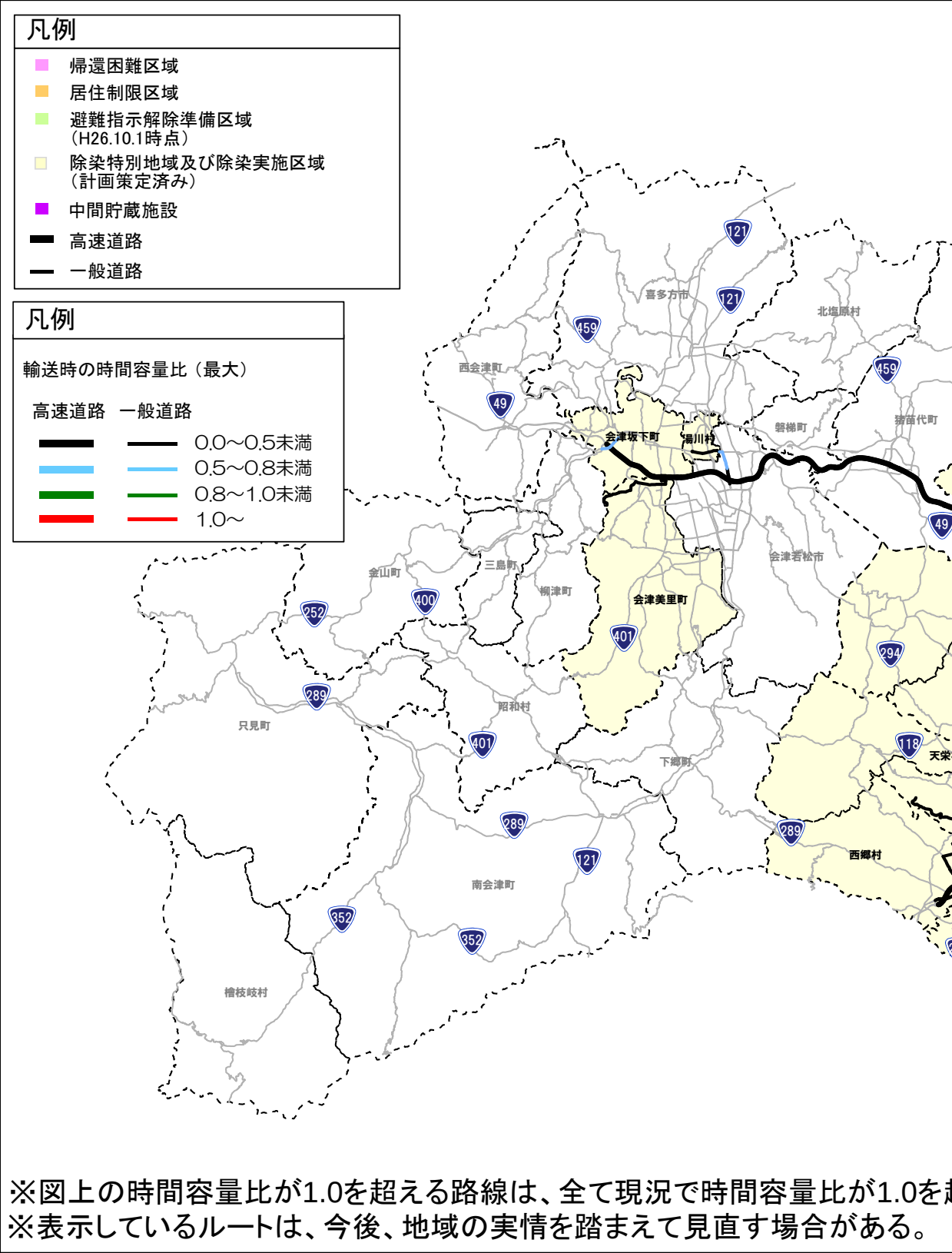
図 7-9 パイロット輸送時「①混雑：輸送車両の時間容量比（最大）」の試算結果
