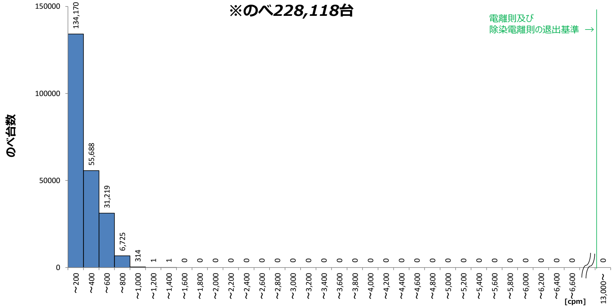
輸送車両のスクリーニング時の最大の表面汚染密度の分布(2020年4月1日～7月31日)
