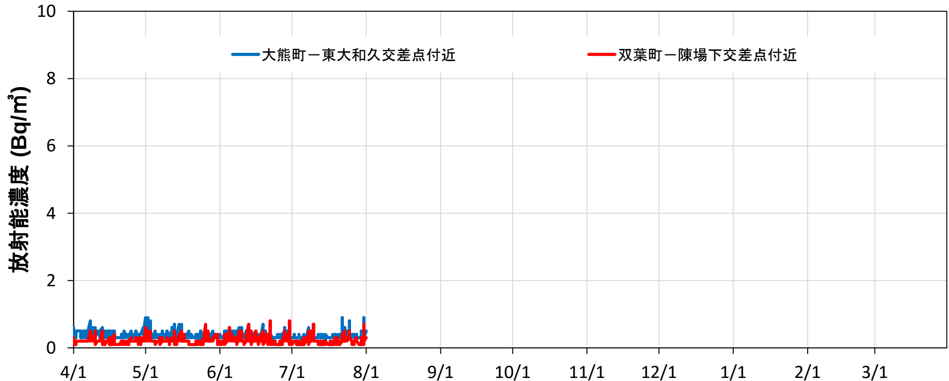
中間貯蔵施設区域境界における大気中の \beta 線の放射能濃度(連続測定) (2020年4月1日～7月31日)
