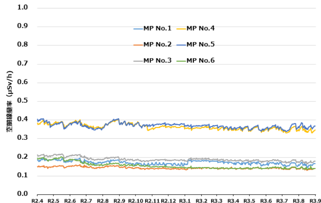
敷地周辺の空間線量率の測定結果
