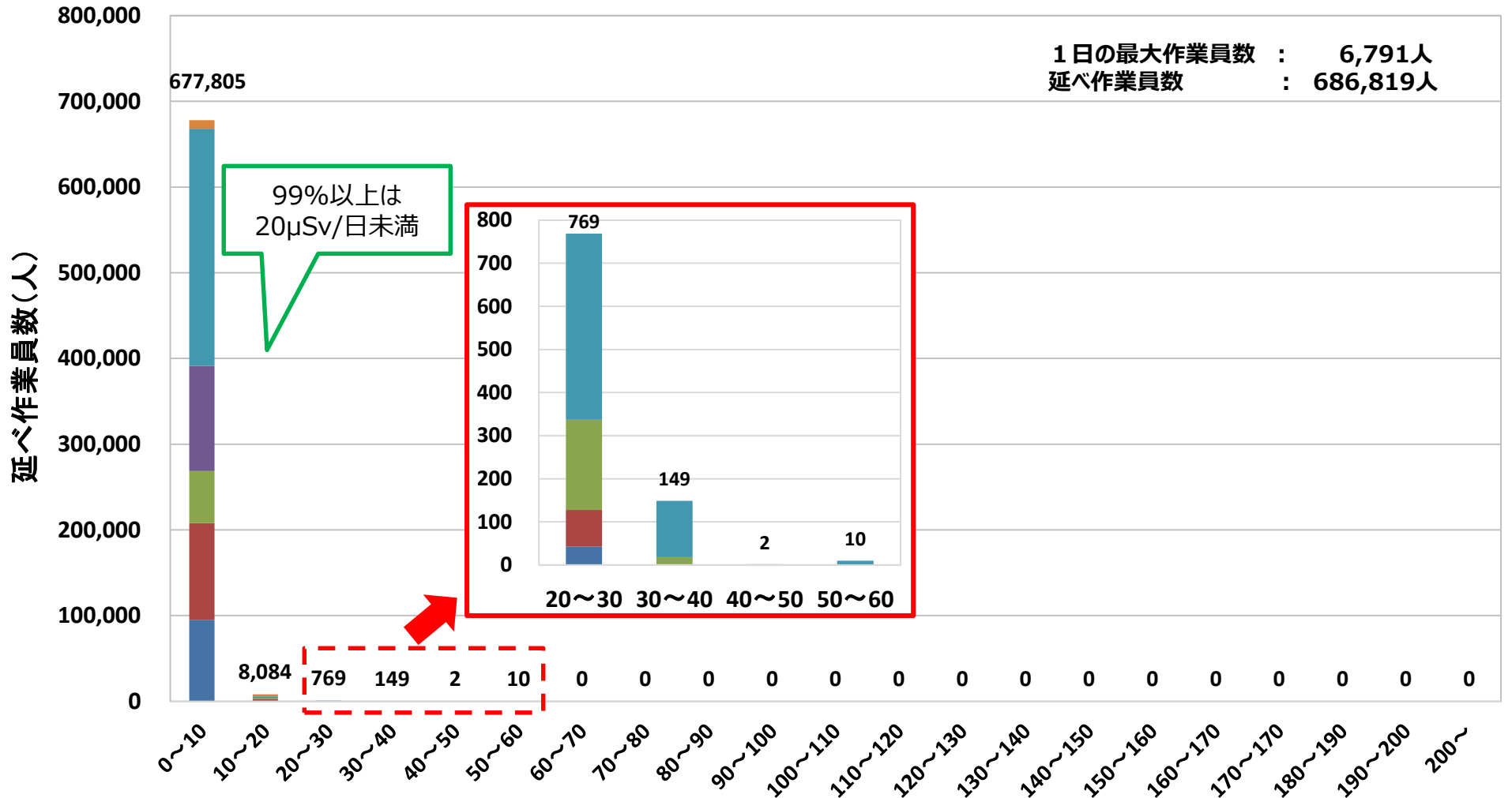
作業員の日次被ばく線量の分布(2021年4月1日～2021年8月31日)
