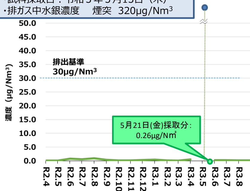
双葉町仮設焼却施設その1 排ガス中の水銀濃度（酸素12%換算濃度）
