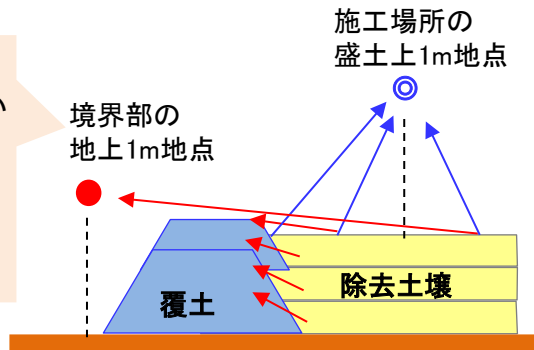
<3層目盛土施工時のイメージ>
