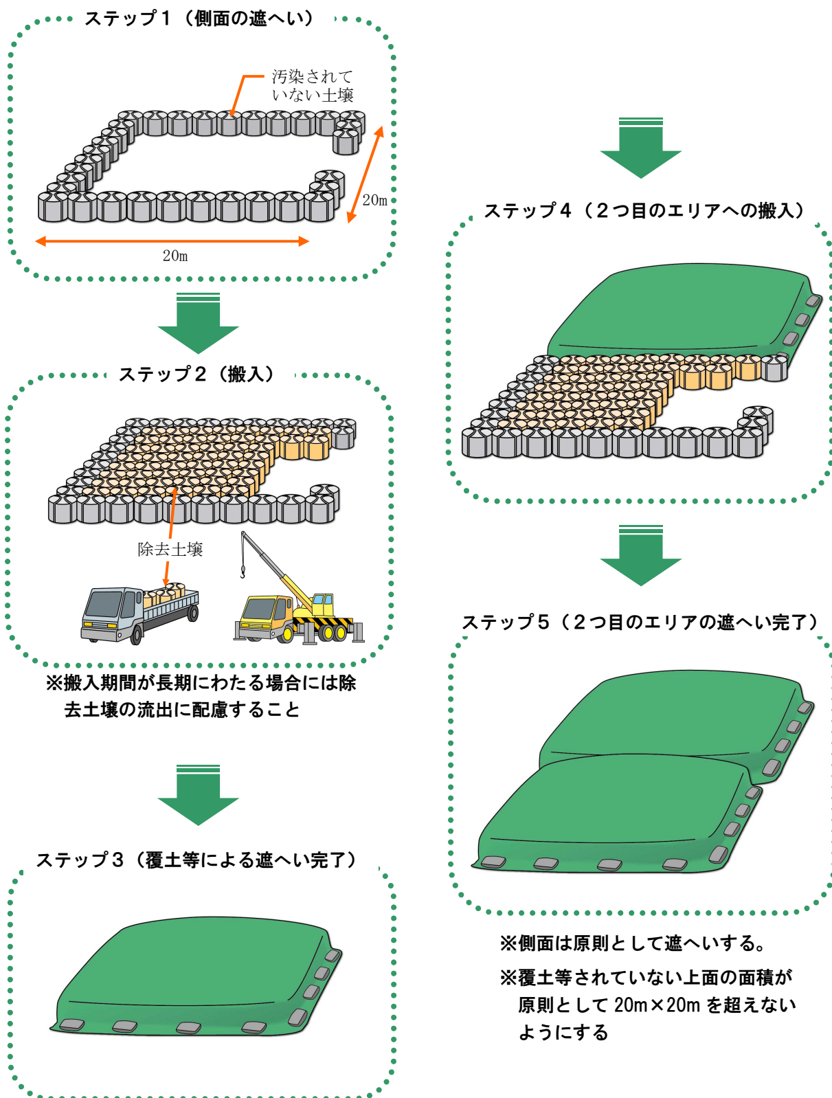
図4-3 大規模な仮置場（側面遮へい）の搬入イメージ
