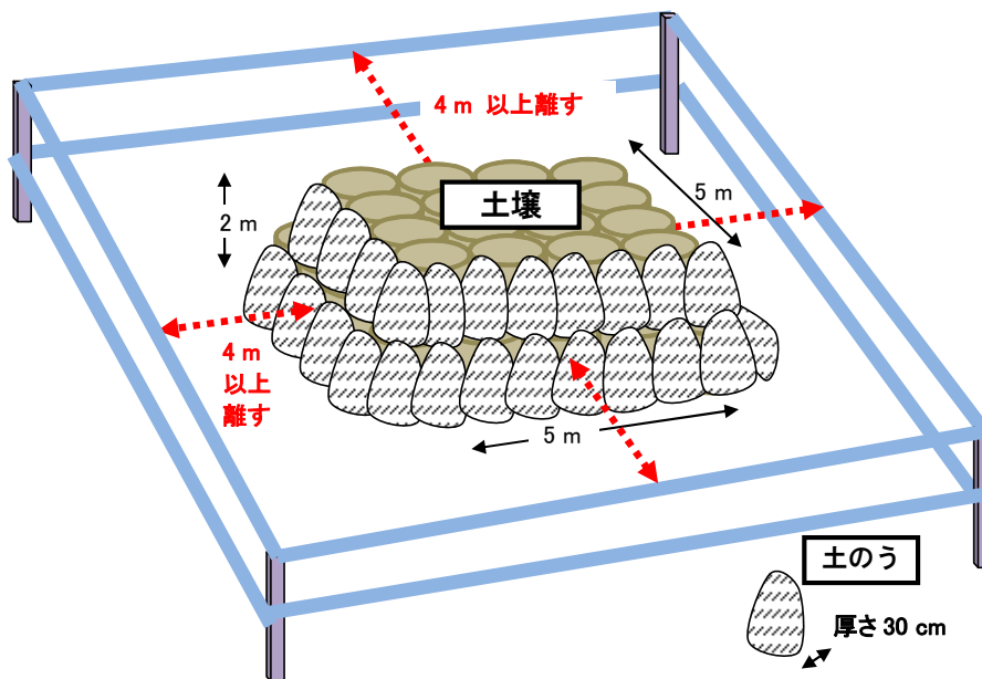
2 万 Bq/kg の除去土壌（縦、横、高さが 5m×5m×2m）に対して側面を土のう（30cm）で遮へいした場合
