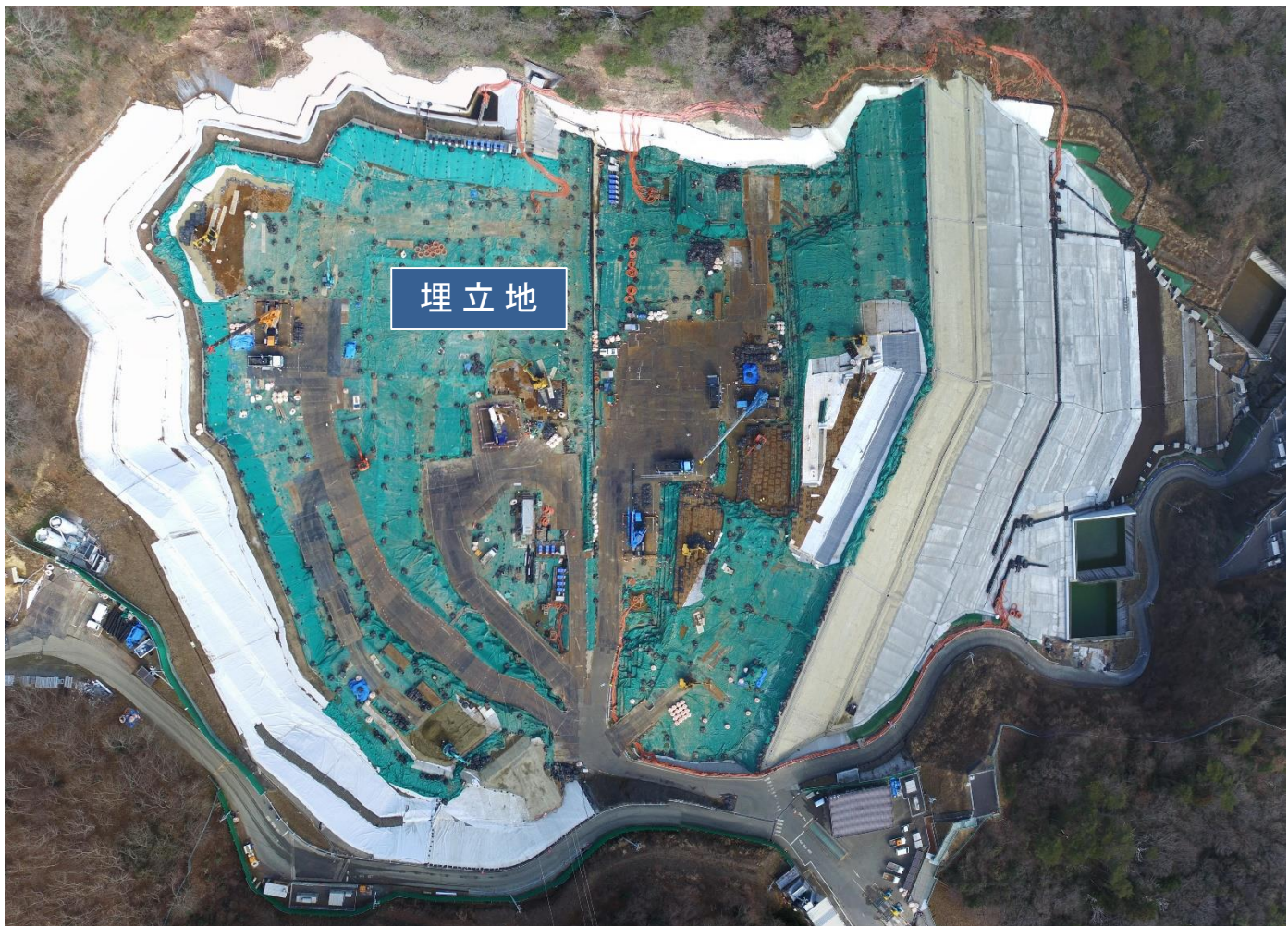
特定廃棄物埋立処分施設（2021年2月1日撮影）
