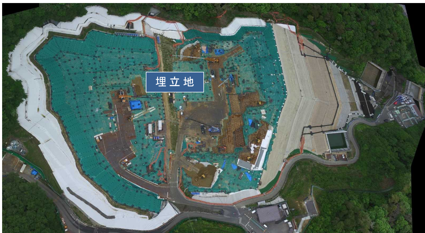
特定廃棄物埋立処分施設 （2020年5月18日撮影）
