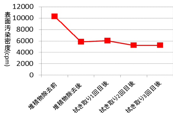
住宅地等の雨樋を対象とした堆積物除去および拭き取りの結果例 (n=3、グラフは平均値)
