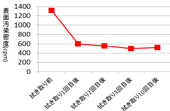
住宅地等の屋根・屋上を対象とした拭き取りの結果例 (n=3、グラフは平均値)
