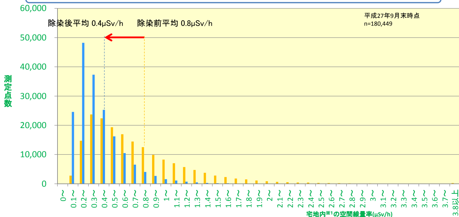
図. 避難指示解除準備区域における除染前後の宅地内空間線量率(1m)の度数分布 (田村市※2、楡葉町※2、川内村※2、大熊町、葛尾村、川俣町、飯舘村、南相馬市、浪江町、富岡町、双葉町)
