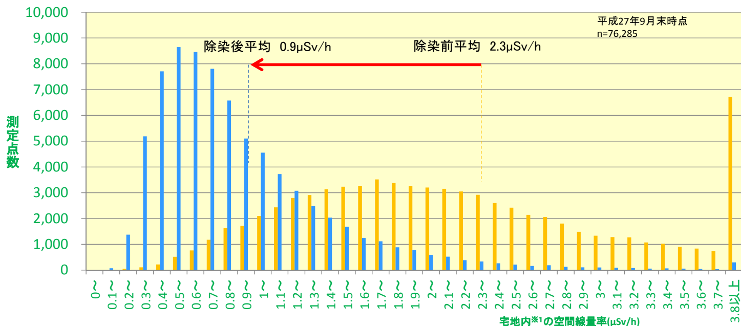
図. 居住制限区域における除染前後の宅地内空間線量率(1m)の度数分布 (川内村※2、大熊町、葛尾村、川俣町、飯舘村、南相馬市、浪江町、富岡町)
