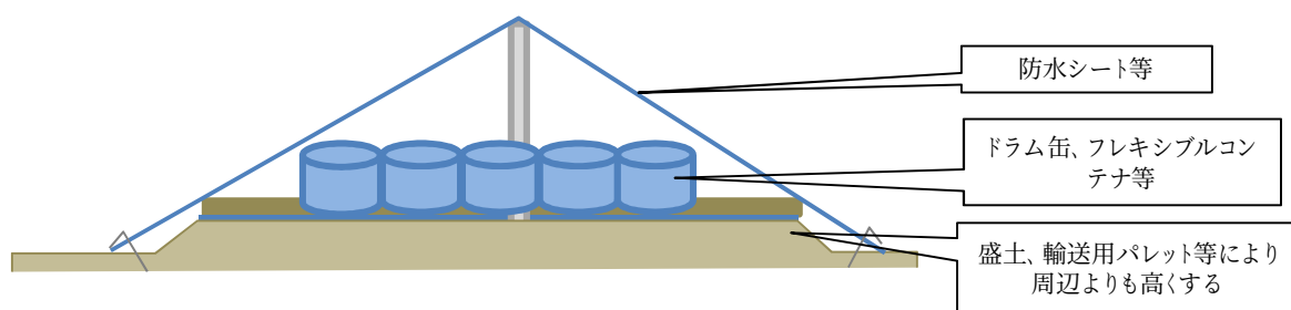
図 2-16 防水シートの屋根を設置した場合の保管（例）
