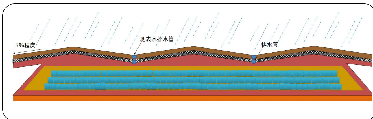
図 5-16 埋立終了時の措置例（２）
