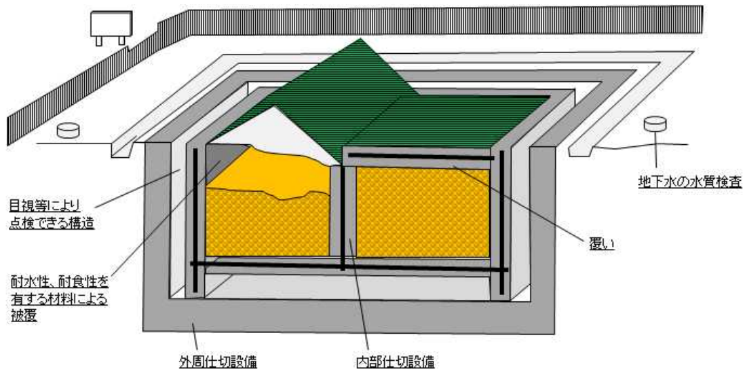
図 5-14 遮断型最終処分場相当の埋立地（例）
