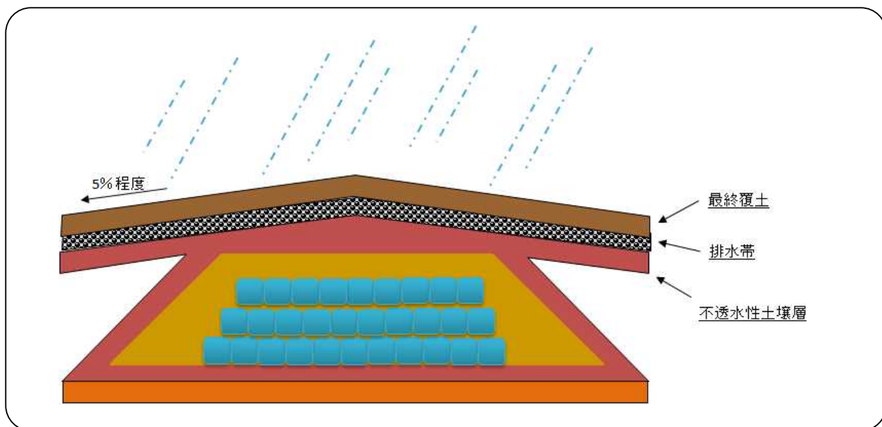
図 5-15 埋立終了時の措置例（１）
