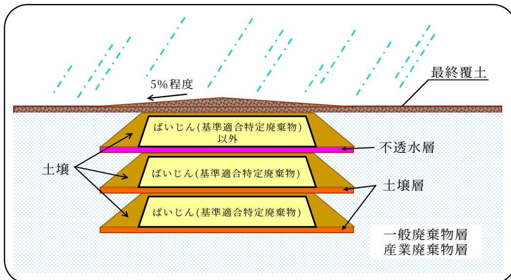
図 5-19 埋立終了時の措置イメージ図（２）
