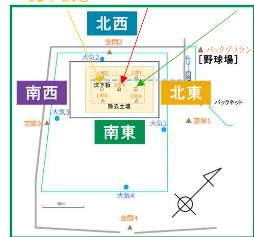
沈下板③ 沈下板② 沈下板①
