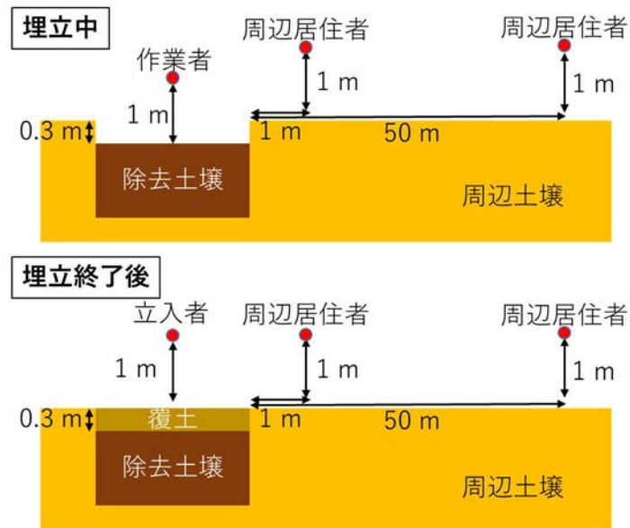
図1 埋立中と埋立終了後の評価体系と評価位置
