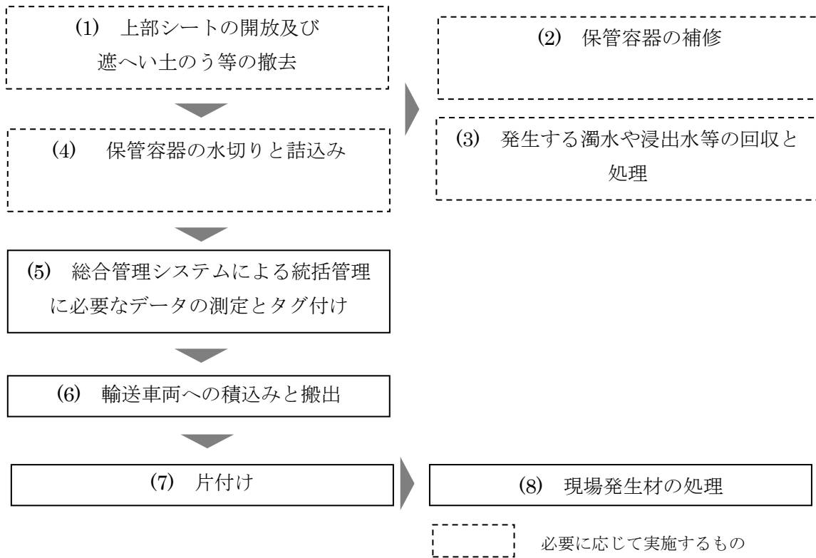
図 2.1.3-1 作業フロー
