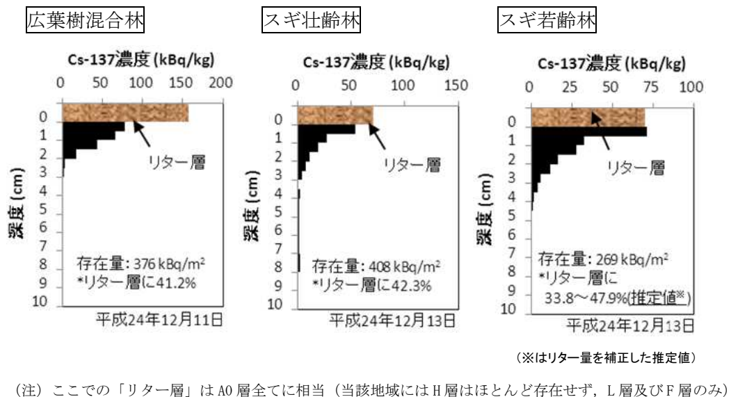
図 2-64 森林における土壌中の放射性セシウム濃度の深度分布
