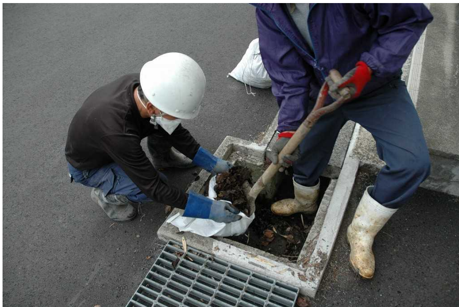
図 2-23 側溝の除染の例（堆積物の除去）
