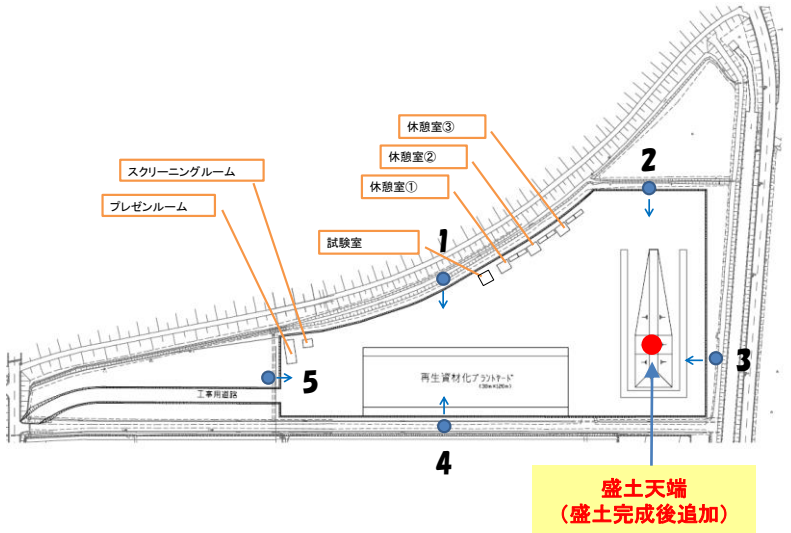
大気中放射能濃度用ダスト採取位置及び吸引方向 (図は2017年8月までの実証ヤード平面図)
