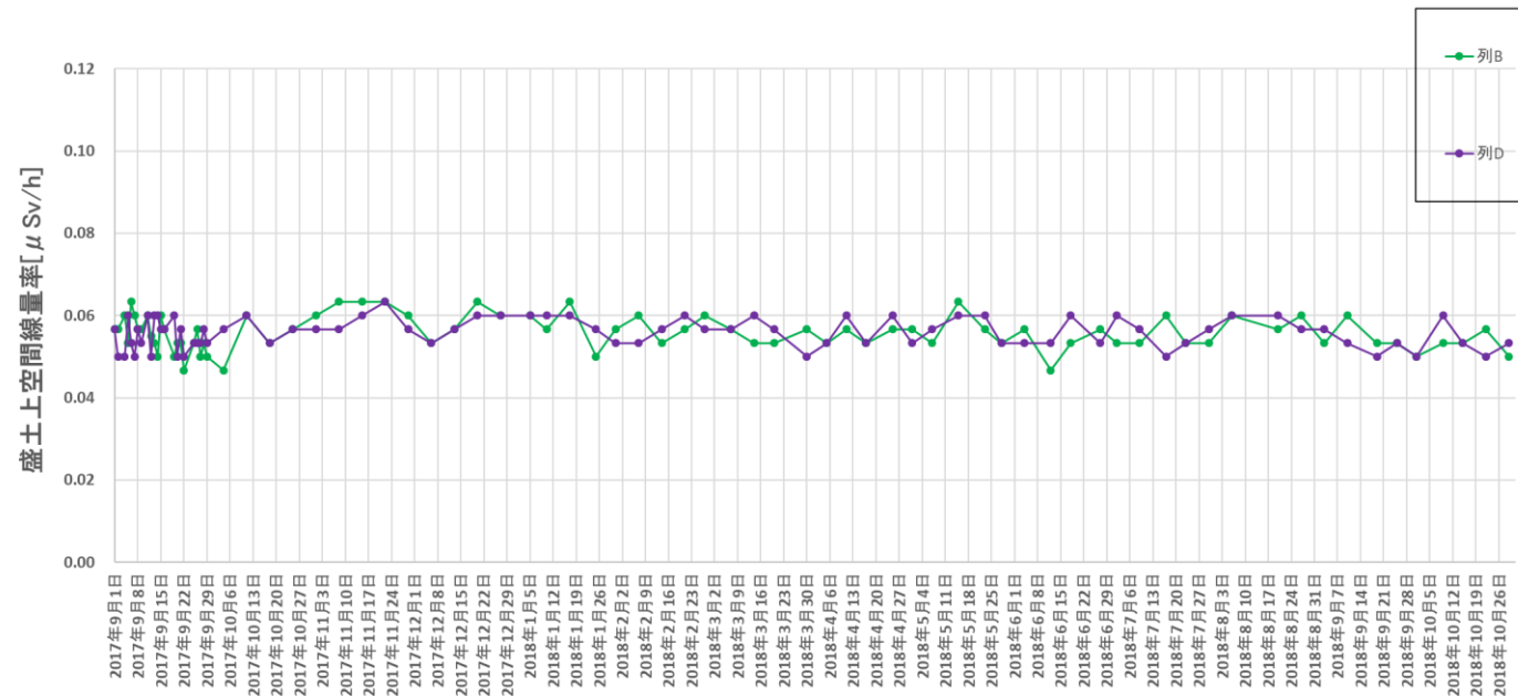
盛土の空間線量率時系列 (列BはNo.7,12,17、列DはNo.9,14,19の平均値)
