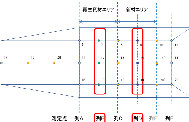
盛土における空間線量率の測定点
