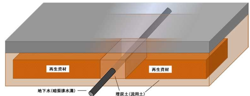
管渠が横断している場合の施工方法の検討例(イメージ)
