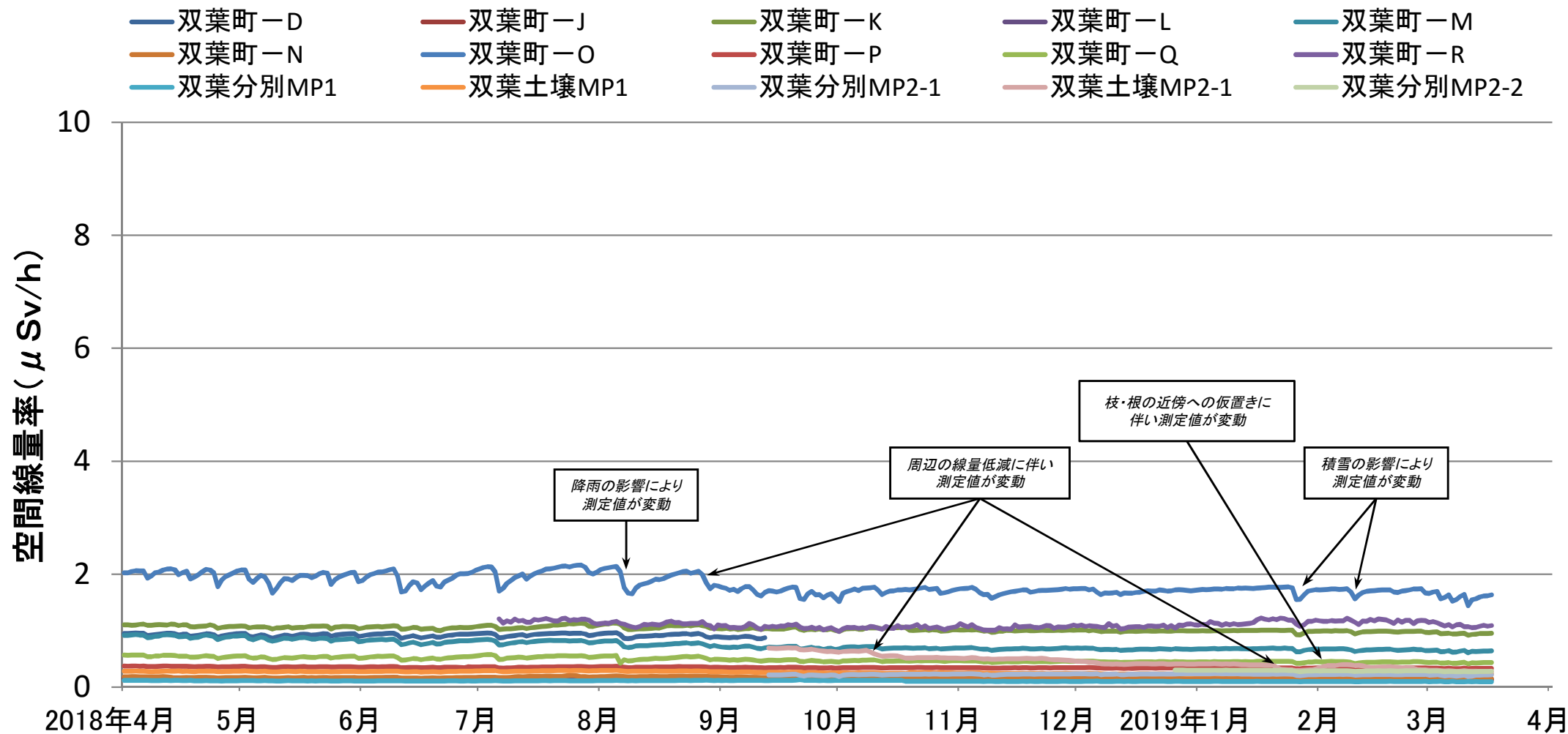
保管場等境界における空間線量率の推移(連続測定)(2018年4月1日～2019年3月17日)
