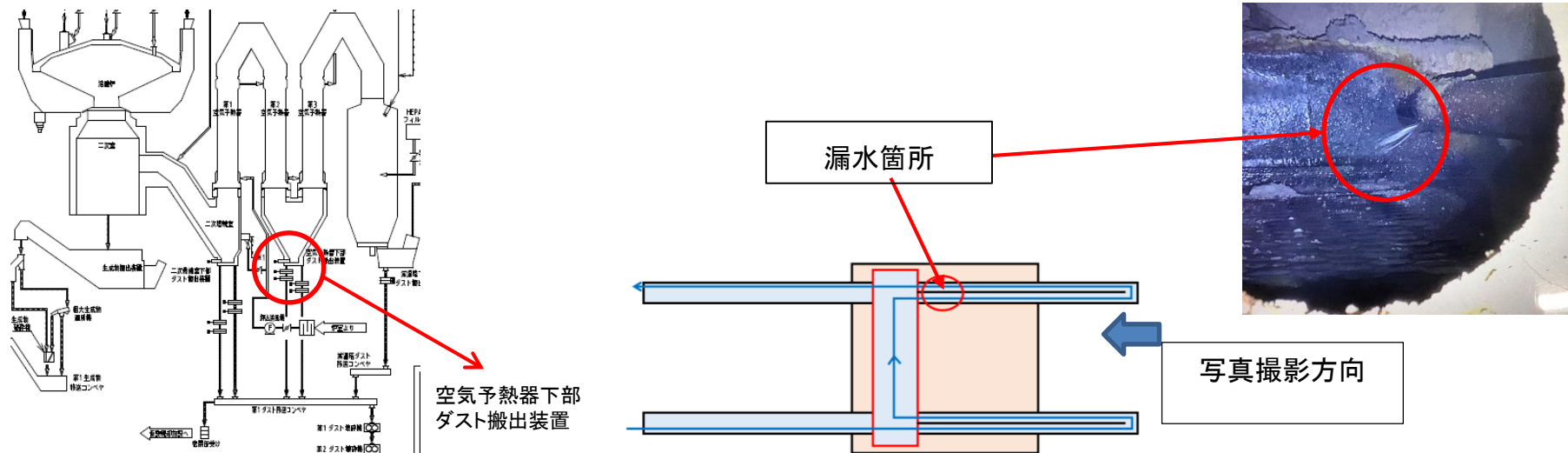
図１ 空気予熱器下部ダスト搬出装置の損傷状況
